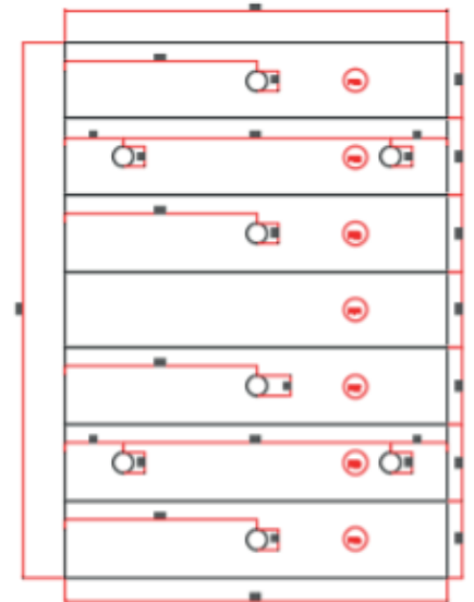
Plafond et réservations diffuseurs
